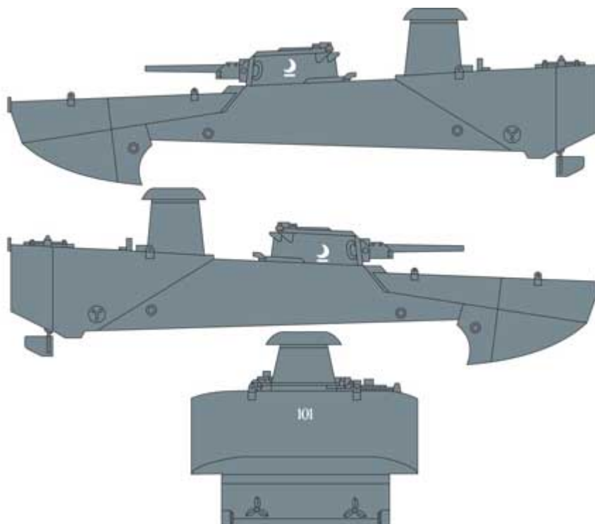
⑦ Typ 2 Ka-mi. Specjalne Siły Desantowe Marynarki. 1944. Type 2 Ka-mi. Navy Special Landing Forces. 1944.
