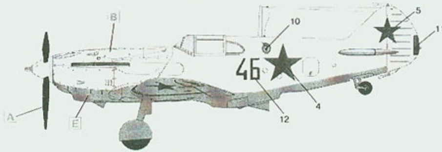
ЛаГГ-3 7-й серии, 3-й ГвИАП ВВС КБФ, район Ленинграда, февраль 1942 г. LaGG-3 series 7, 3th GvIAP (Guard Fighter Regiment) of Baltic Fleet Air Force, Leningrad area, February 1942
