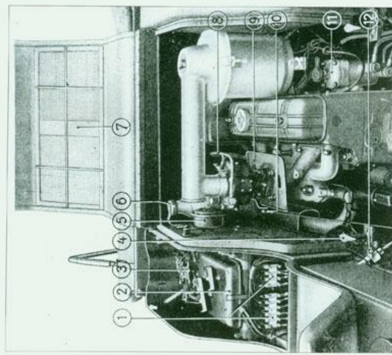
Engine compartment from the front, sowing box closed • Ansicht Motorraum von vorne, Motorhaube hochgeklappt, Saatfächer geschlossen; 1-Sicherungen - Fuses, 2-Sammeler - Collector, 3-Schnecken - Sowing chains, 4-Rechter Motorhaubehalter - Right bonnet mount, 5-Horn, 6-Ölfasche - Oil bottle, 7-Motorhaube - Bonnet, 8-Kraftstoffleitung - fuel pipe, 9-Vergasertropfbüchse - Carburetor collector, 10-Drosselklappenhebel - throttle lever, 11-Ölspartfilter - Oil filter, 12-Rechter Kraftstoffhahn - Right fuel cock.
