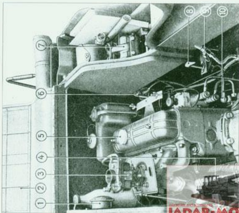
Engine compartment from the front, sowing box opened • Ansicht Motorraum von vorne, Motorhaube hochgeklappt, Saatfächer geöffnet; 1-Horn - Horn, 2-Motorhaube - Bonnet, 3-Schnecken - Sowing chains, 4-Rechter Motorhaubehalter - Right bonnet mount, 5-Horn, 6-Ölfasche - Oil bottle, 7-Motorhaube - Bonnet, 8-Kraftstoffbehälter - fuel pipe, 9-Vergasertropfbüchse - Carburetor collector, 10-Linker Kraftstoffhahn - Left fuel cock, 11-Luftleitung zur Öldruckwarmlampe - Cable guide to oil pressure warning light.
