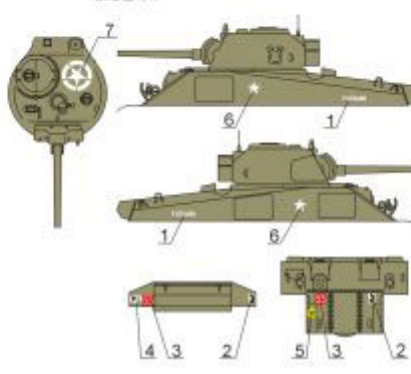
D Sherman V 24 Pułk Ułanów 1 Dywizja Pancerna, Holandia, 1944. Sherman V 24th Lancers Regiment, 1st Polish Armoured Division, Holland, 1944.
