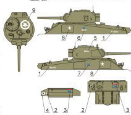
F Sherman V Doser, 24 Pułk Ułanów 1 Dywizja Pancerna, Niemcy, 1945. Sherman V Doser, 24th Lancers Regiment, 1st Polish Armoured Division, Germany, 1945.
