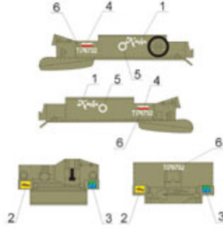
☒ Universal Carrier nr 1. 25 Pułk Ułanów Wielkopolskich, 5 Kwatera Dywizji Piechoty Litwów, Wilno, sierpień 1945. Universal Carrier nr 1. 25th Wielkopolski Lancers Regiment, 5th Infantry Division, Lwów, Italy, August 1945.
