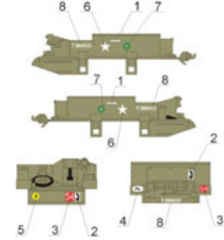
☒ Universal Carrier nr 8. 4 batalion ckm, 4 Dywizja Piechoty, Szkocja, 1945. Universal Carrier nr 8. 4th MG Battalion, 4th Infantry Division, Scotland, 1945.
