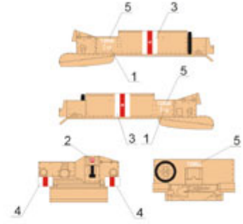
[K] Universal Carrier mk I, Samozbrojna Brygada Strzelców Karpackich, Gzasko, styczeń 1942. Universal Carrier mk I (Polish) Independent Carpathian Rifle Brigade, Gzasko, January 1942.
