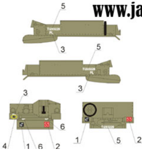
C Universal Carrier mk I. 24 Pułk Ułanów, 1 Dywizja Pancerna, Szkocja, 1943. Universal Carrier mk I. 28th Lancers Regiment, 1st Armoured Division, Scotland, 1943.
