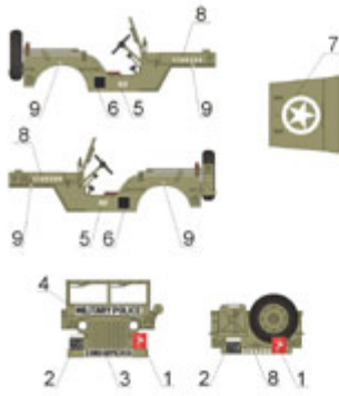
D Willys MB: 3 Batalion Strzelców Karpackich, 3 Dywizja Strzelców Karpackich, Włochy, 1945 Willys MB: 3rd Carpathian Rifle Battalion, 3rd Carpathian Rifle Division, Italy, 1945
