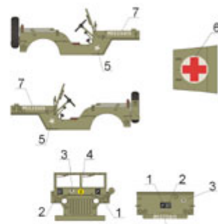
I Willys MB: Kompania artylerii lekkiej, 1 Samodzielna Brygada Spadochronowa Bersebrück, Niemcy 23.08.1945 Willys MB: Light Artillery Company, 1st Independent Parachute Brigade, Bersebrück, Germany, 23.08.1945
