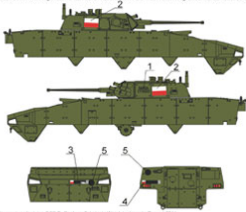
5. Rosomak z oddziału OSS-D: Centrum Szkolenia Wojsk Lądowych, Polesie 2011 / Rosomak with OSS-D turret: Land Forces Training Center, Polesie 2011
