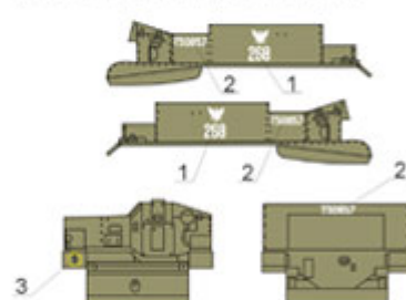
13. Universal Carrier mk I, 5 Pułk Czołgów Ciężkich, Niemcy, kwiecień 1945. Universal Carrier mk I, 5th Heavy Tank Regiment, Germany, April 1945.
