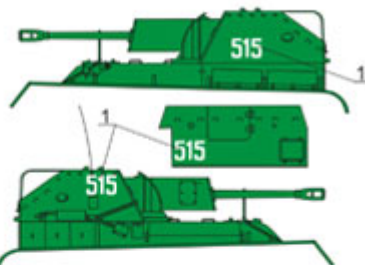
12. IS-2m, 3 kompania, 4 Samodzielny Pułk Czołgów Ciężkich, Rejon Berlina, kwiecień 1945. IS-2m, 3rd Company, 4th Independent Heavy Tank Regiment, Berlin area, April 1945.
