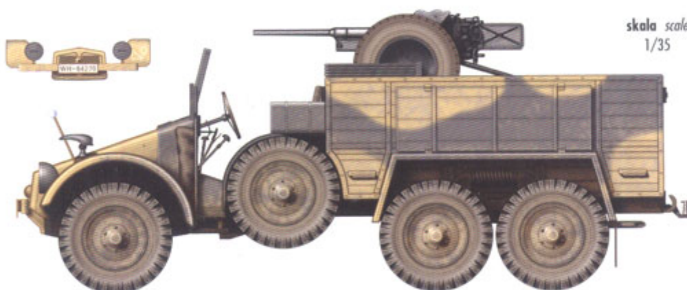
Krupp L 2 H 143 (6x4) Kfz 70 z armatą 3,7 cm Pak 35/36 z nieustalonej jednostki, front wschodni, jesień 1942 roku. Krupp L 2 H 143 (6x4) Kfz 70 with 3.7cm Pak 35/36 AT gun from unidentified unit on Eastern Front in Autumn 1942.
