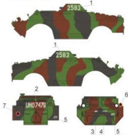
2. BRDM-2 M66. 2 Pulk Rozpoznawczy, 2011 r.
