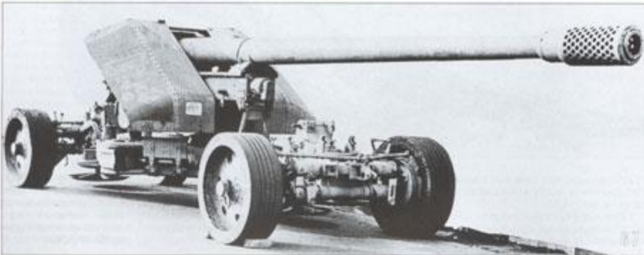
67, 68. 128-мм противотанковое орудие PaK 44 фирмы Крупп в транспортном (фото 67) и боевом (фото 68) положении (АСКМ).
