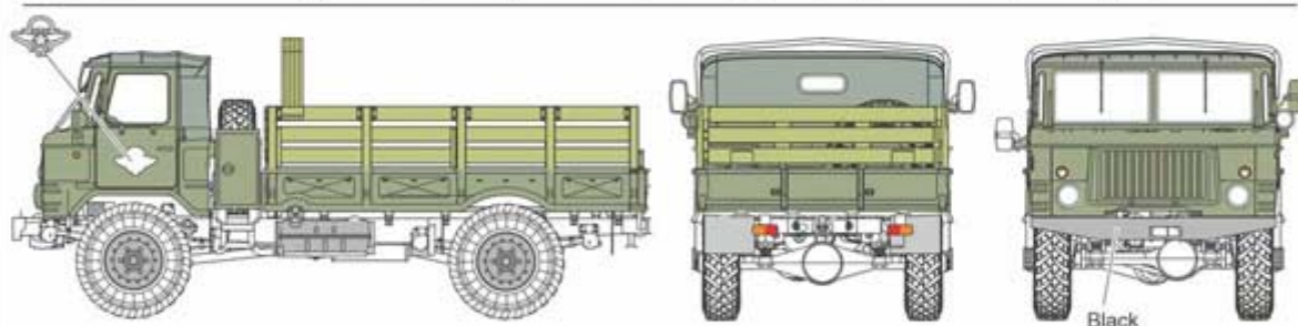
2t AWD military truck model 66B. Soviet Union paratroopers. Standard painting. Mid 1970-th. Soviet khaki-green. 2т вантажівка ГАЗ-66Б. Радянські повітряно-десантні війська. Стандартне забарвлення. 70-ті роки. Радянський хаки.
