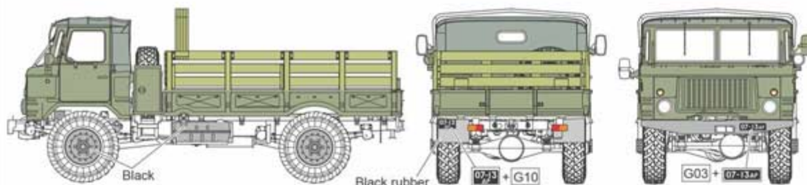
2t AWD military truck model 66B. Soviet VDV (paratroopers). Mid 1970th. Soviet khaki-green. 2т вантажівка ГАЗ-66Б. Радянські повітряно-десантні війська. 1970-ті роки. Радянський хаки.
