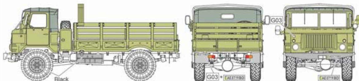
2t AWD military truck model 66B. Private collection. Light Green (Close to FS 13670). Mid 201x. Ukrainian Dnepr Region. 2т вантажівка ГАЗ-66Б. Приватна колекція, Україна. Номери Дніпровського регіону. Салатово-зелений. 201x.
