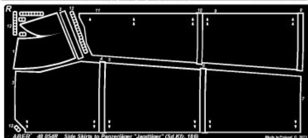
48 054 Side skirts for Panzerjäger Jagdtiger (Sd.Kfz. 186) (TAMIYA model)
